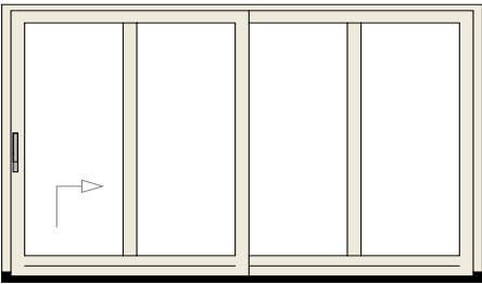
HSP-2Q ⑤⑥⑦ ■ ▶ hefschuipui 2-delig, quadra
