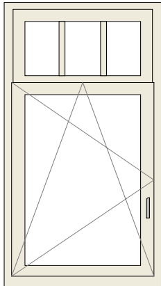
Amsterdamskozijn Opplakroede Type A, 32 mm
