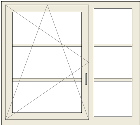
Draai-kiepraam met zijlicht Opplakroede, type A, 32 mm
