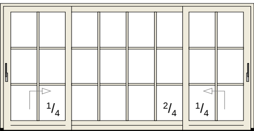
HSP-3K glasverdeling 1/4, 2/4 en opplakroede type A, 32 mm
