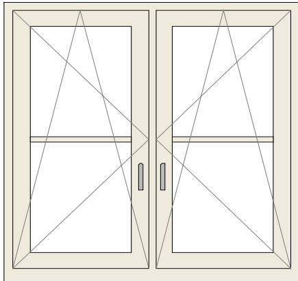
2x Draai-kiepraam Opplakroede, type A, 32 mm
