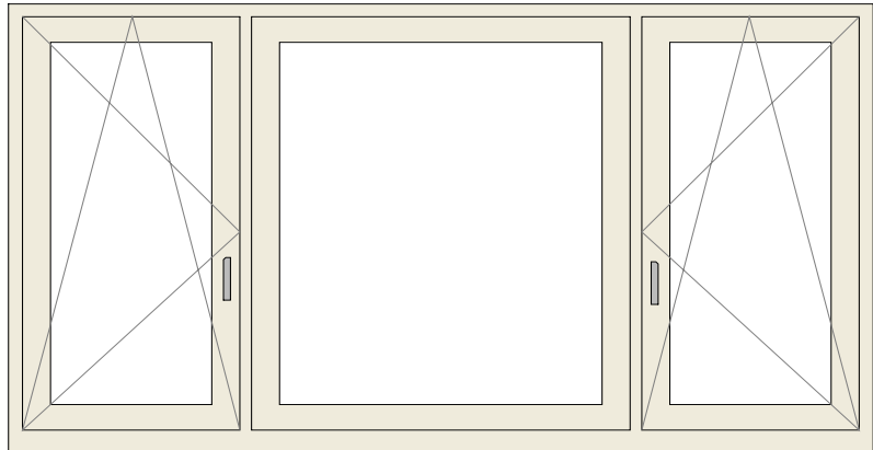
2x Draaikiep-raam en vast raam Opplakroede, type A, 32 mm
