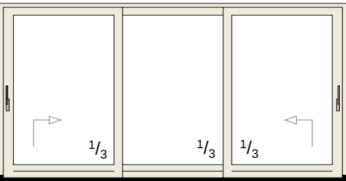
HSP-3K ⑤⑥⑦ ■▶ hefschuifpui 3-delig, 2 buitendeuren schuivend
