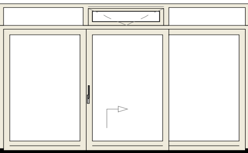
HSP-3G3 bovenlicht met uitzetraam
