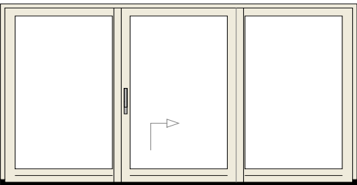
HSP-3G2 ⑤⑥⑦ ■ hefschuifpui 3-delig, symmetrisch
