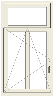
Amsterdamskozijn Glasdelende roede Type H, 75 mm
