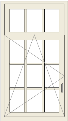
Amsterdamskozijn Opplakroede Type A, 32 mm
