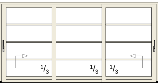
HSP-3K glasverdeling 1/3, 1/3 en opplakroede type A, 32 mm
